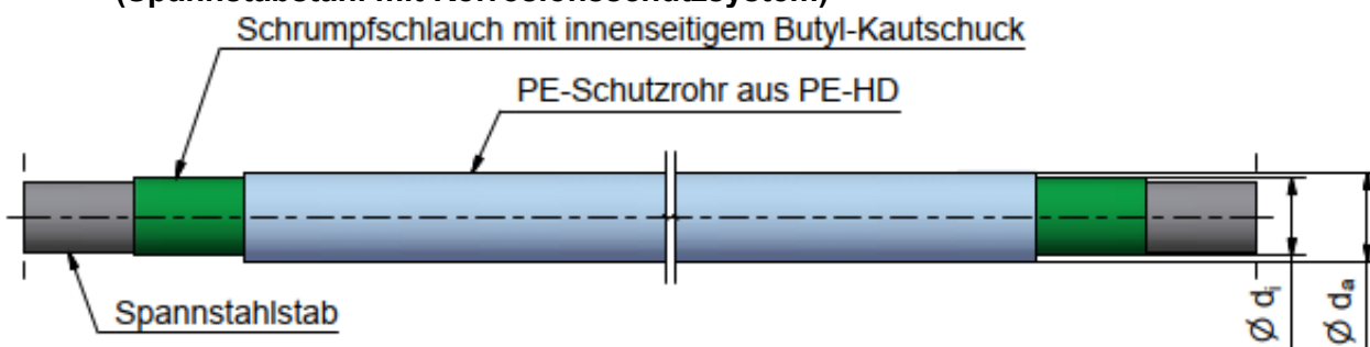
Bild 3: Schematische Darstellung des Zulassungsgegenstandes nach Abschnitt 1.3 (Spannstabstahl mit Korrosionsschutzsystem)
