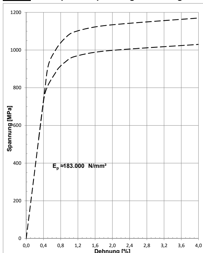
Bild 2: Prinzipieller Spannungs-Dehnungsverlauf
