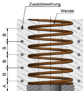
Prinzipskizze Lo3 - Lo9
