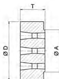
Lochscheibe
