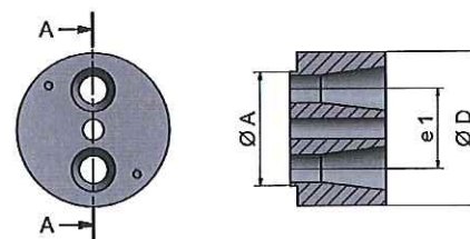
Lochscheibe LoE-2
