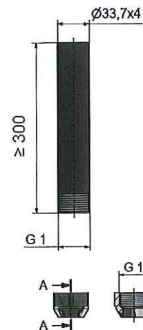
Ankerstützen mit Konusmutter
