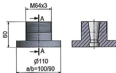
Ankerkopf LoE-1
