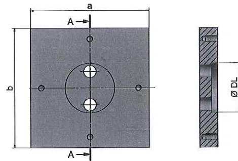
Lochscheibe LoE-2
