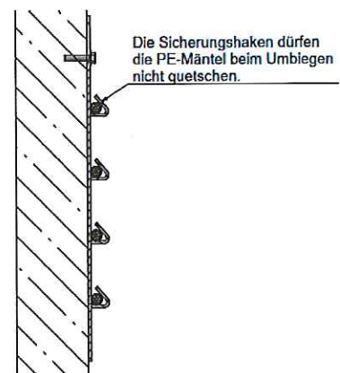
nach der Montage (Schnitt A-A)
